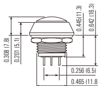
12-mm Type: F/PB
